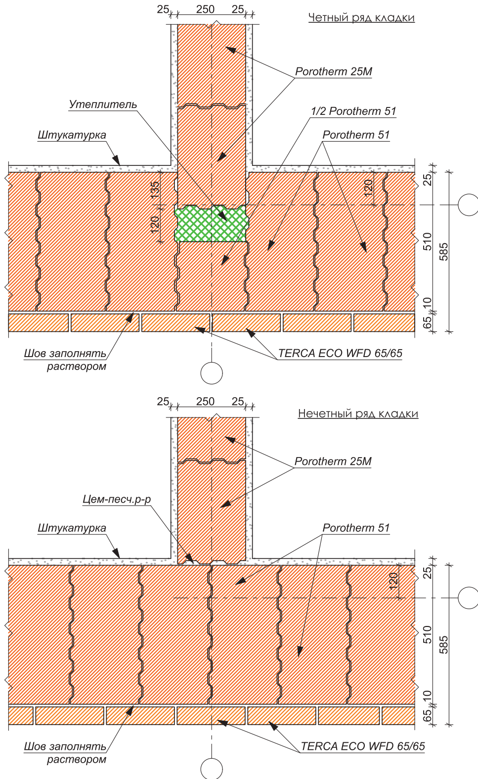
УЗЕЛ СОПРЯЖЕНИЯ НАРУЖНОЙ СТЕНЫ, ТИП 2, ИЗ POROTHERM 51 С ВНУТРЕННЕЙ СТЕНОЙ ИЗ POROTHERM 25M
