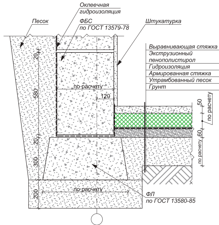
Фундаментная подушка
