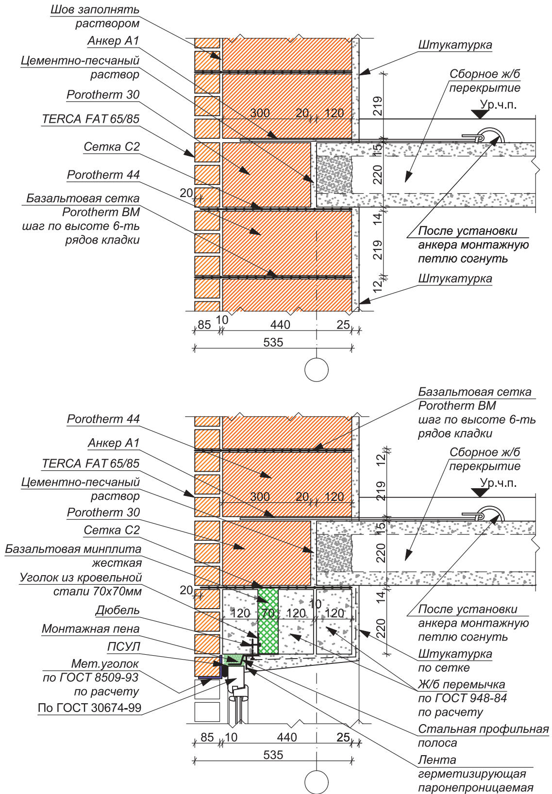
СТЕНА, ТИП 2. УЗЛЫ (POROTHERM 44)
