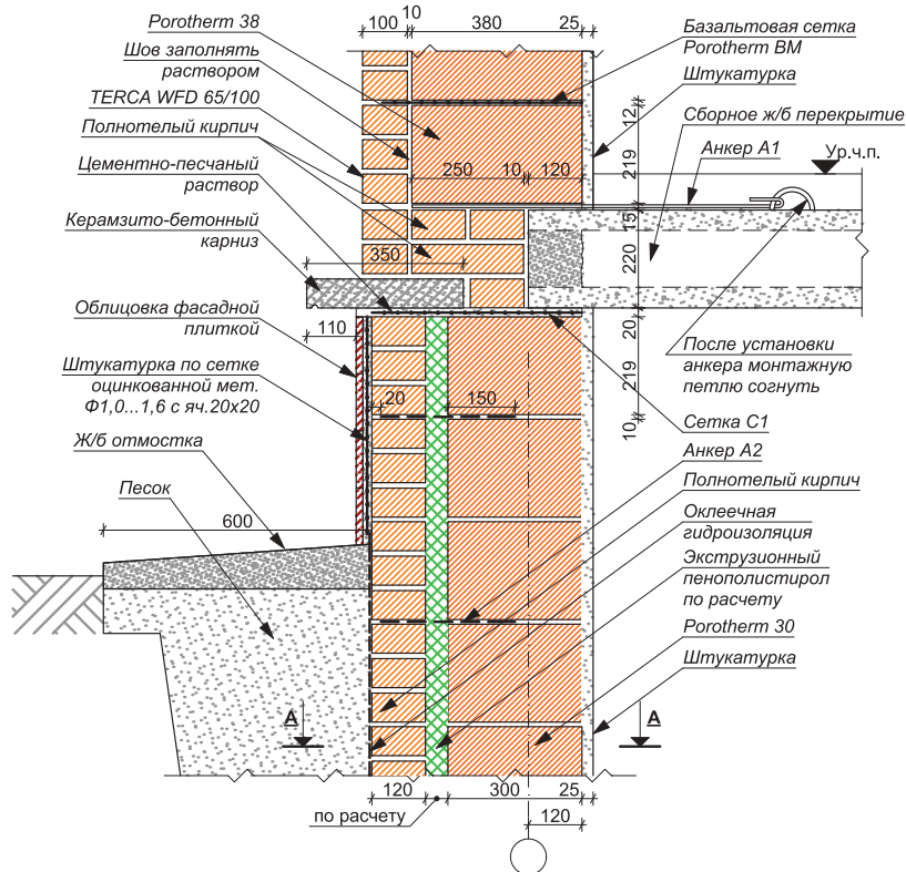
СТЕНА, ТИП 2. ОТАПЛИВАЕМЫЙ ПОДВАЛ. СБОРНЫЙ ФУНДАМЕНТ (POROTHERM 30, POROTHERM 38)
