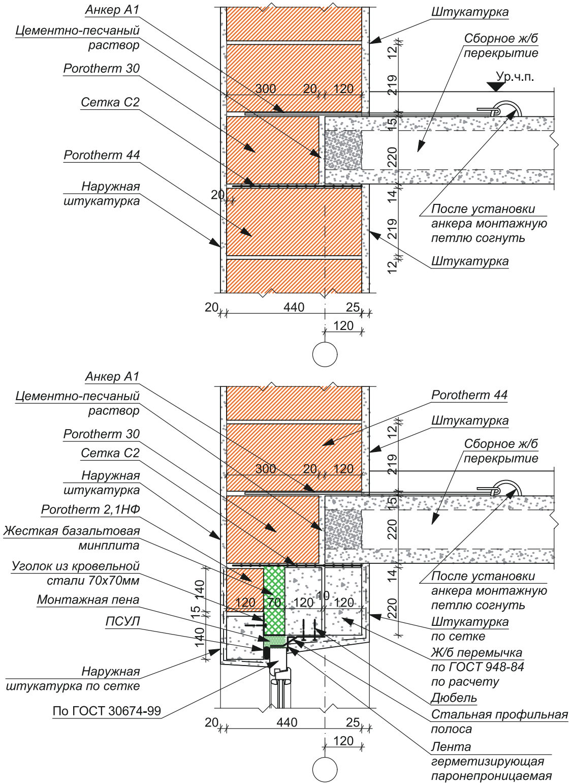
СТЕНА, ТИП 1. УЗЛЫ (POROTHERM 44)
