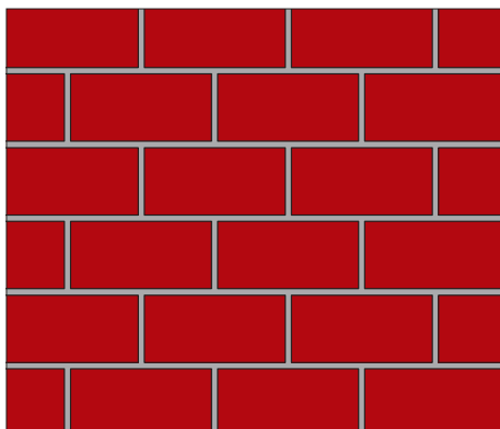
Половинная перевязка
