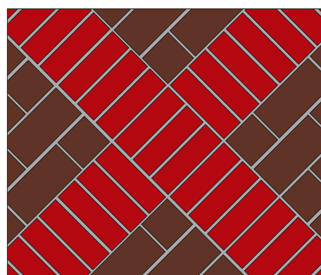
Половинная перевязка в полкамня с осевым размыканием
