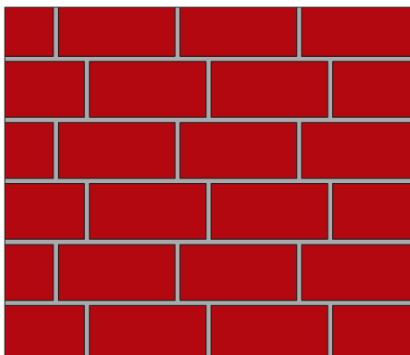
Трёхчетвертная перевязка
