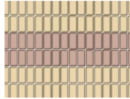
«Паркетная» укладка на тычок
