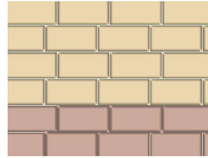
Трехчетвертная перевязка
