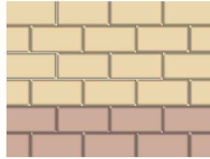
Половинная перевязка
